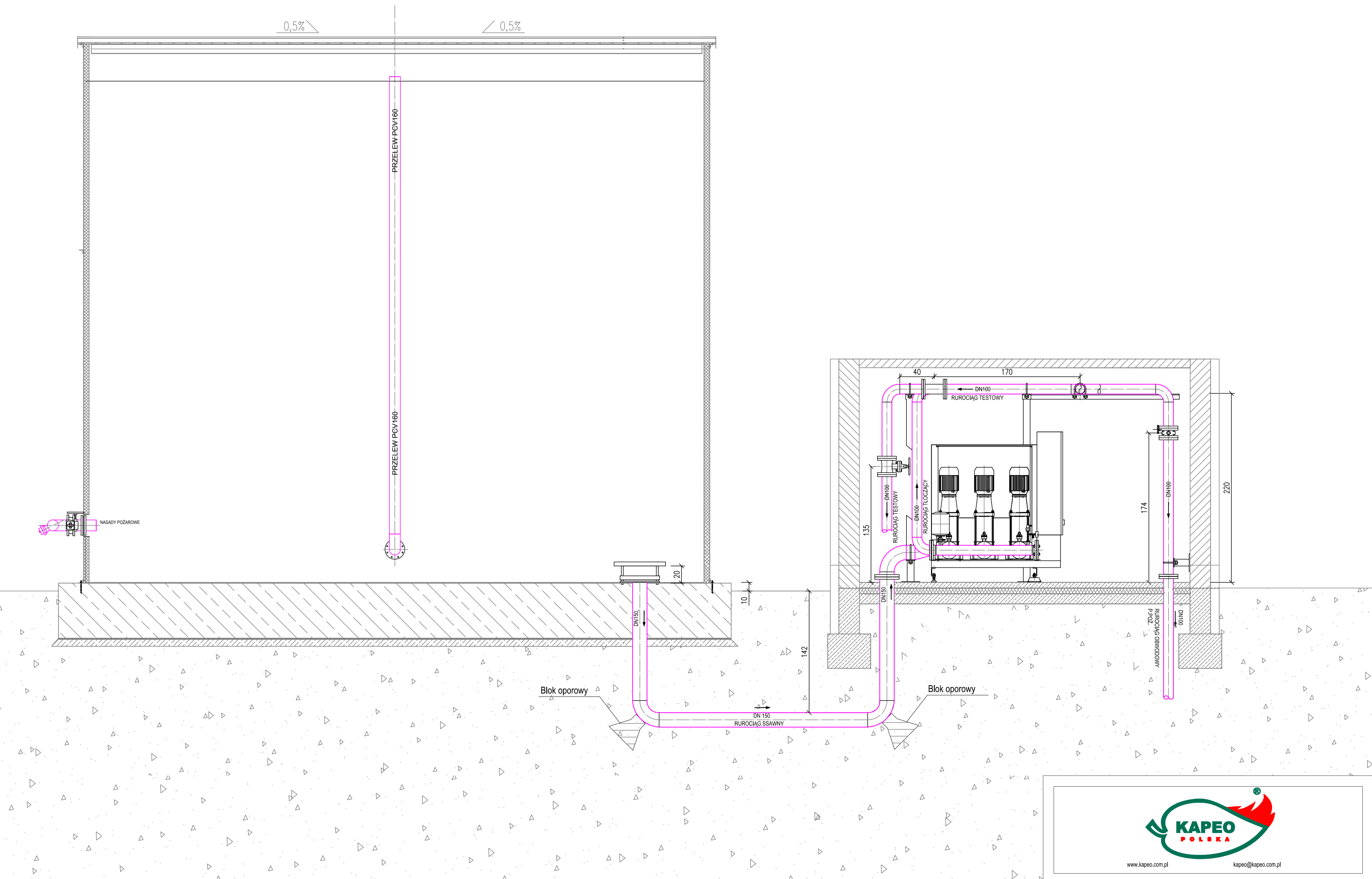
PRZEKRÓJ A-A
